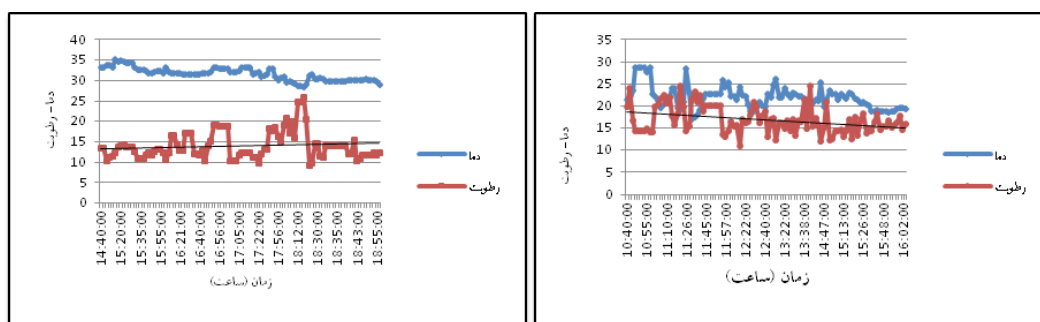
نمودار ۳ و ۴: رابطه میان دما، رطوبت و زمان (ساعت) در محله علی‌قلی‌آقا (سمت راست: فصل زمستان، سمت چپ: فصل تابستان)
